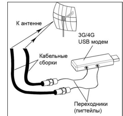
Примеры установки и подключения антенны к оборудованию
