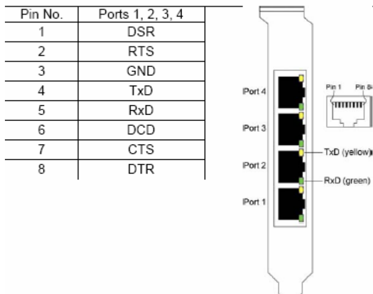
RS-232
